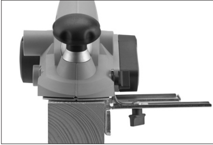
Kenar posasının monte edilmesi.
